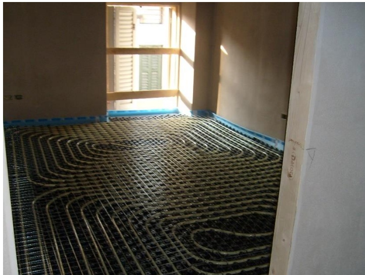
Palazzo Paletta Dai Prè -Verona - Abitazione privata: realizzazione di impianto a pannelli radianti a pavimento in edificio storico
